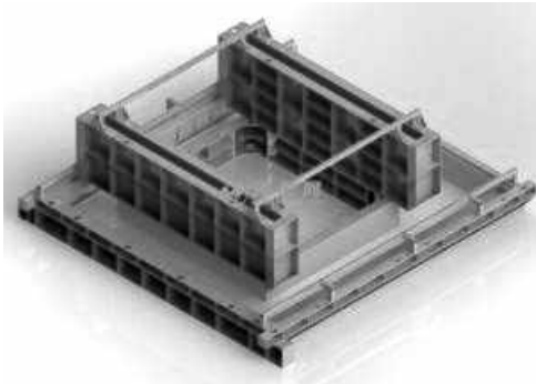
图1 装配式预制飘窗模具
