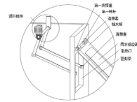
图2 调节组件示意图
