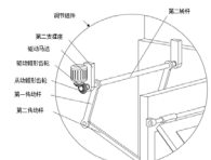
图3 调节组件结构图
