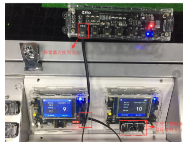
图1 报警器节点及传感器模块
