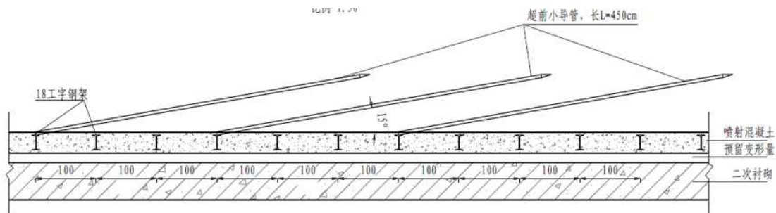
图1 超前小导管布置详图
