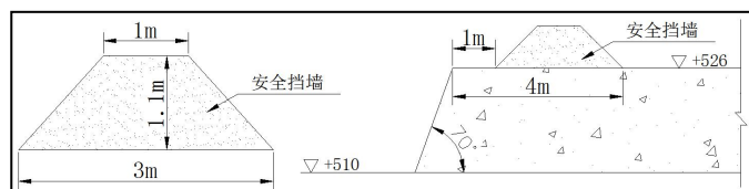
工作面安全挡墙典型横断面示意图
