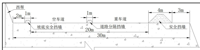
主干道路典型横断面示意图
