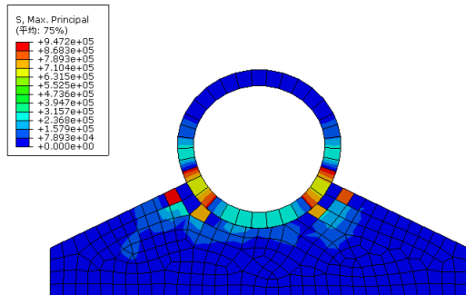
图 3 工况 1 最大主拉应力分布图 (Pa)
