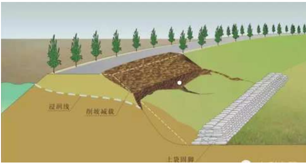
图2.1 堤防位移坍塌加固图
