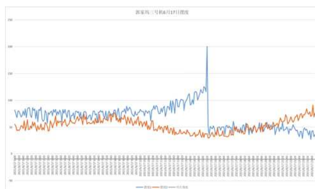
郭家坞三号机6月17日摆度
