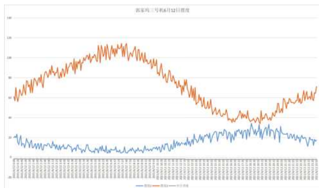
郭家坞三号机6月12日摆度
