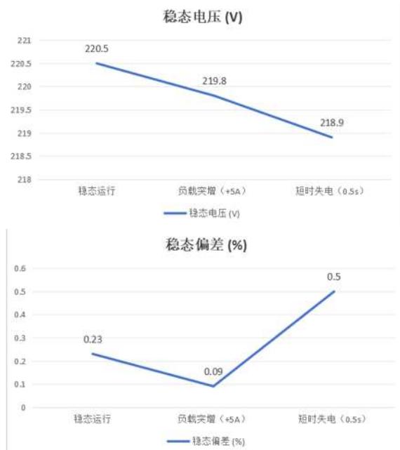
图 1 稳态电压与稳态偏差变化
