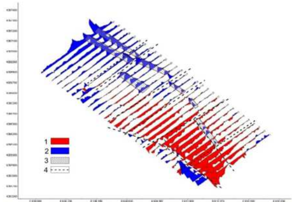
图 3.ΔT, nT 图, M1:100000 ;1-ΔT 负值, 2-ΔT 正值, 3-« 磁铁矿砂岩 », 4- 断口。
