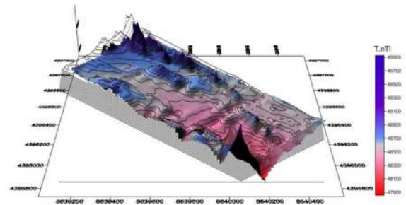
图 2.T, nT1 三维动力学线图, M1:100000。
