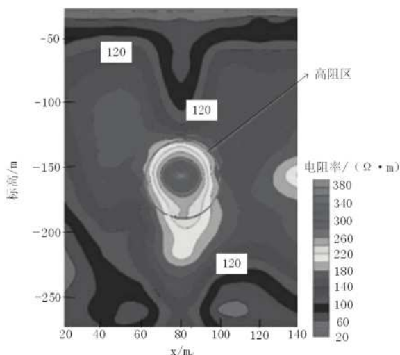
图2 中心回线法电阻率的断面结果图
