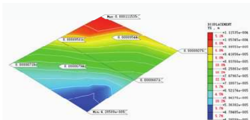
图10 绿地公园建造后底板结构竖向位移云图
