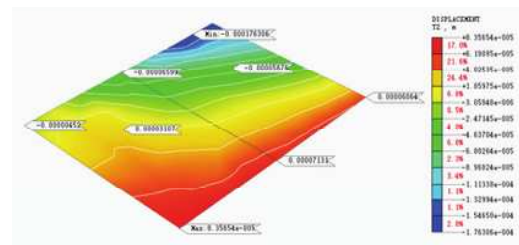
图11 市政道路建造后隧道结构竖向位移云图
