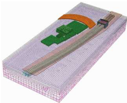
图3 新建工程与铁路2号隧道的相互关系
