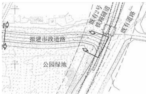
图1 拟建工程与2号隧道的平面关系图
