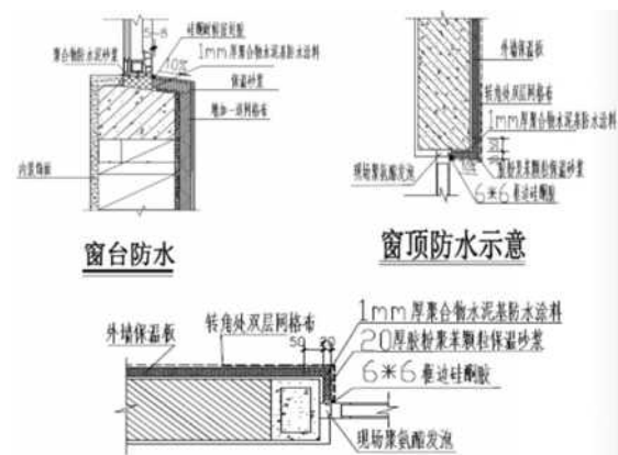
图1 窗侧板防水
