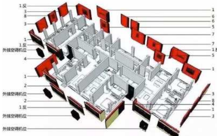
图3 施工鸟瞰图
