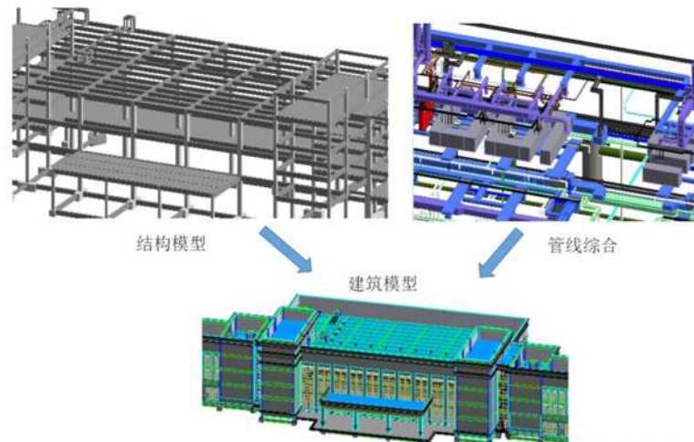
图2 BIM项目设计可视化示意图
