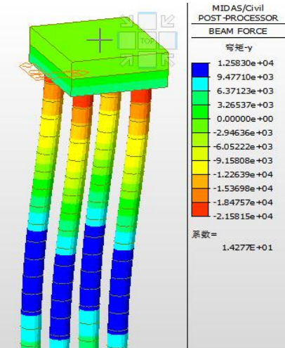
图 5 防撞墩受力计算结果（弯矩）
