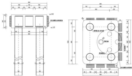
图 3 防撞墩构造图
