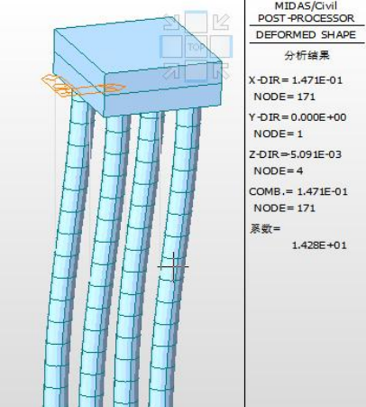
图 6 防撞墩受力计算结果（位移）
