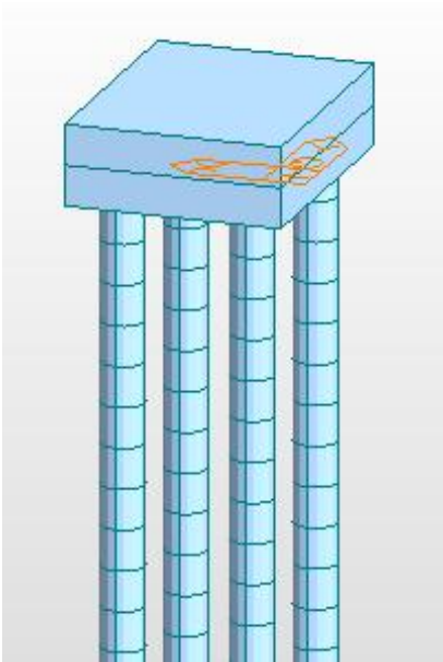
图 4 防撞墩受力计算模型（模型渲染）
