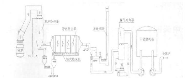
图一：干法除尘系统工艺流程图
