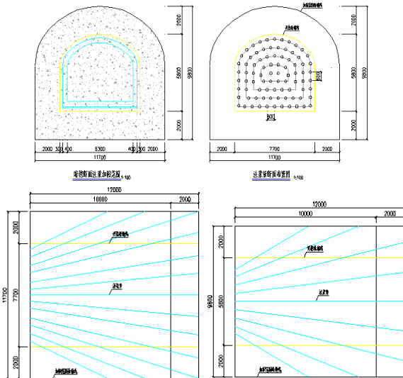
图 1 浆加固范围及注浆管纵、断面布置图
