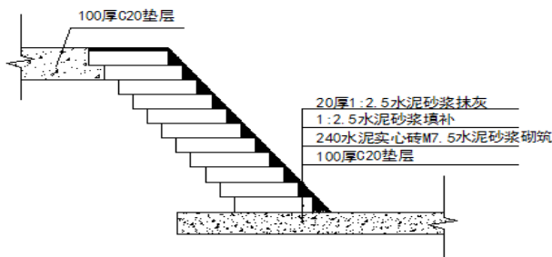
图3 砖胎膜内侧抹灰图
