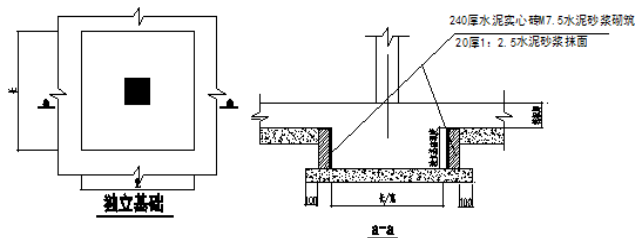
图1 独立基础砖胎膜示意图
