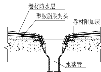
水落管处防水做法大样图
