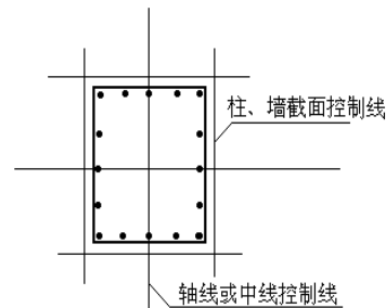
柱、墙模板放线示意图
