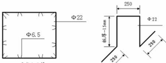
图7 钢筋制作绑扎图
