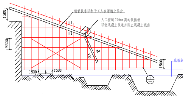
图5 泵管架布置图
