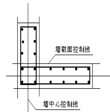
柱、墙模板放线示意图
