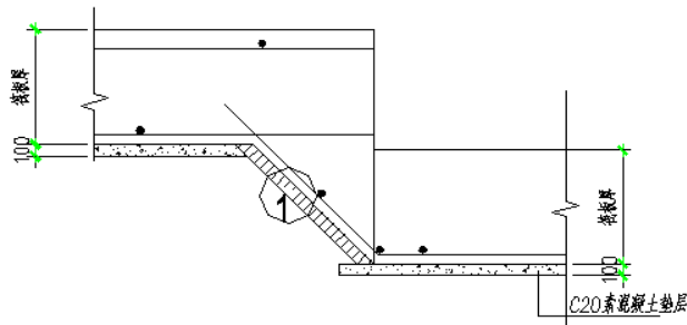
图2 高低跨砖胎膜示意图
