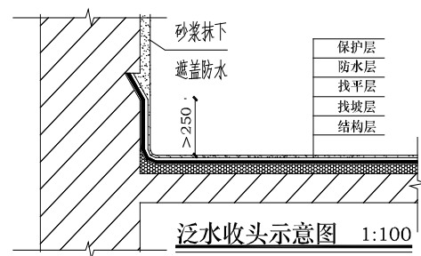
图9 泛水收头示意图
