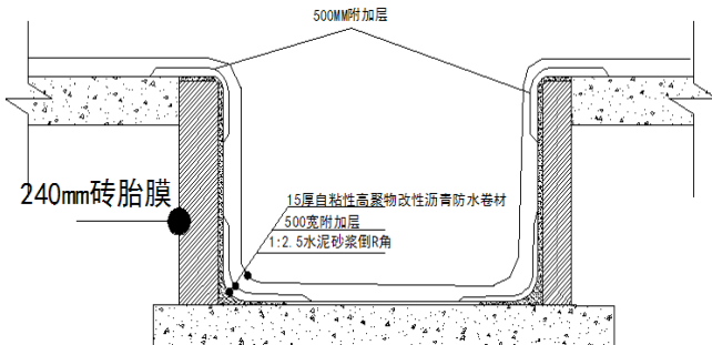
图4 阴阳角抹灰图
