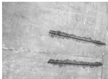
图2 房屋混凝土楼板露筋
