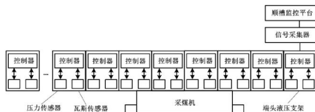
图1 采煤机速度控制系统结构图
