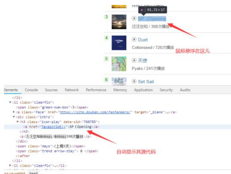
图4 自动显示源代码
