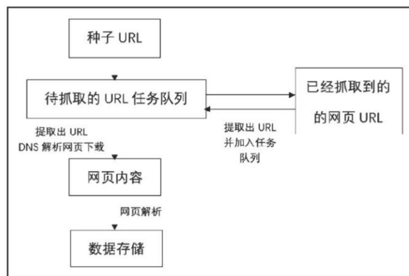
图 1 爬虫的基本流程
