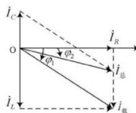
图2 补偿前后向量关系示意图
