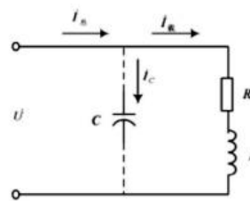
图1 等效电路示意图
