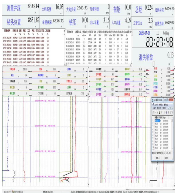
图1 立压、悬重异常抓拍
