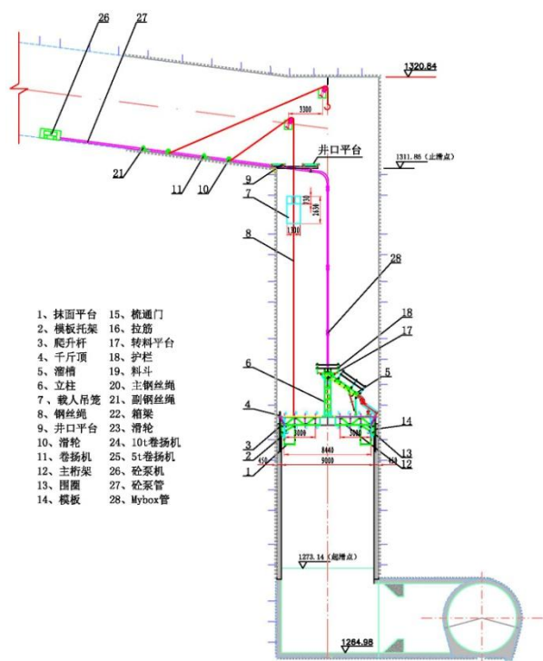
图1 滑模施工图
