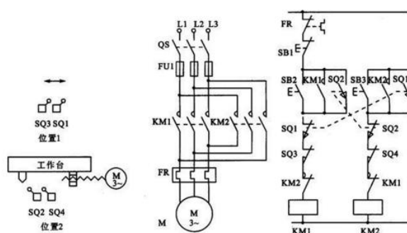
图1 电气自动化控制设备原理图
