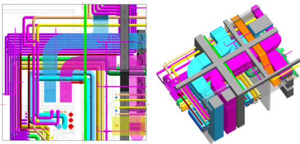
十二层复杂位置 BIM 模型
