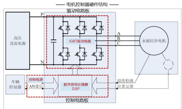
图 2-8 电机控制器硬件结构
