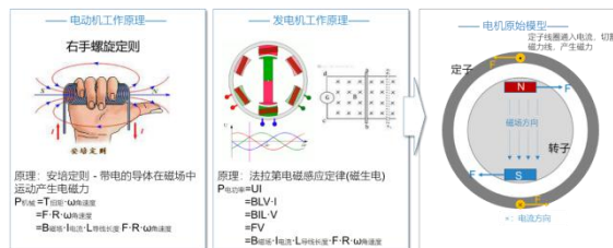
图 2-5 电机系统工作原理
