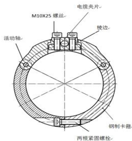
图1 井控用快速电缆固定装置
