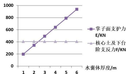
图 17 水囊体厚度对掌子面稳定性的影响
