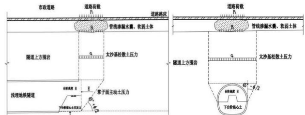
图14 管线渗漏下地铁隧道掌子面稳定性简化计算模型
