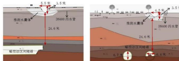
图 2 某地铁区间地面塌陷剖面图
