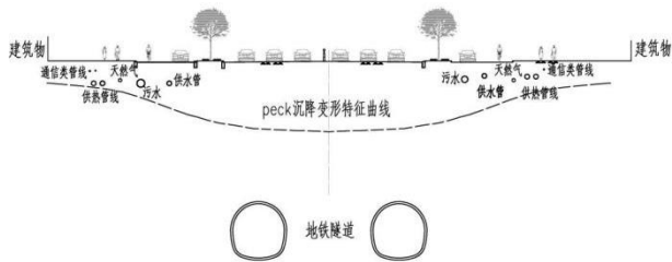
图12 典型地铁区间与管线位置关系图
