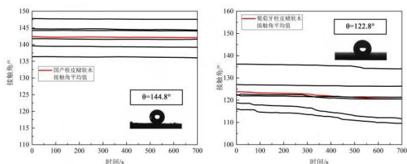
图 1 两种产地软木接触角
