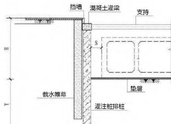
图3 柱列式灌注桩排桩平面示意图
