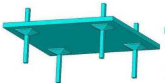
图4 带柱帽的无梁楼盖
