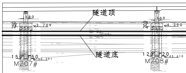
图2 项目桥梁工程与地铁10号线区间隧道相对位置关系示意图
