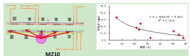
图7 车站段桩基施工空间影响效应(以MZ10#墩柱桩基为例)
