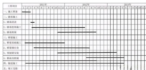
图1 施工进度表
