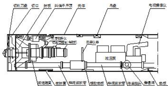
图 2-1 顶管机构造图
