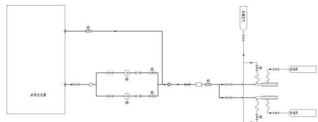
喷水系统图
