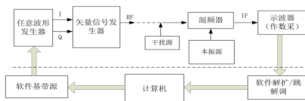
图 1 装置组成框图
