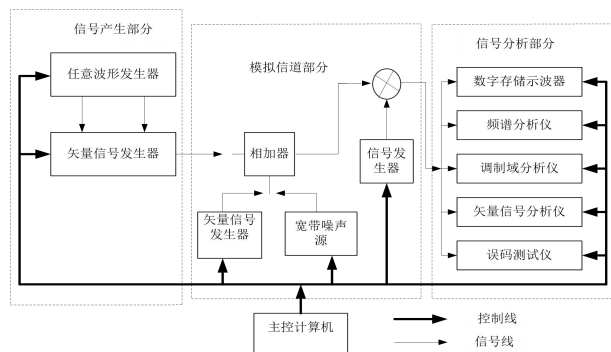
图 8 扩跳频抗干扰系统自动测试平台工作原理框图
