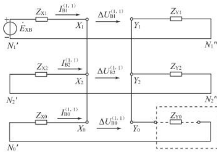
图4 相断线时复合序网图
