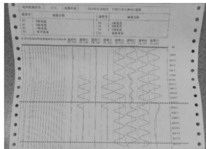
图3 线路故障波形图
