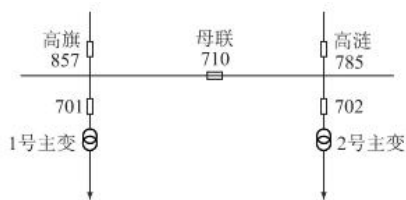
图1 主接线图
