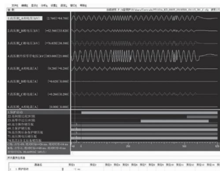
图2 1号主变故障波形图
