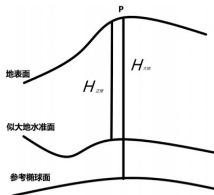
图2 大地高、正常高、正高的关系
