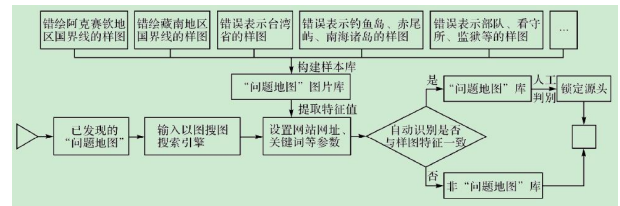
图2 基于样本库的以图搜图自动识别流程图
