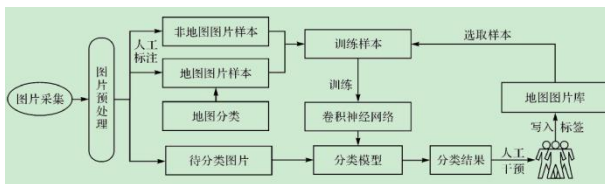
图1 基于卷积神经网络的图片识别流程图
