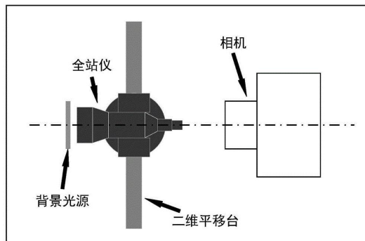
图2 全站仪相机示意图
