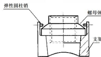
图2 XX7715-2002 桶形螺母
