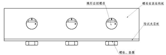
图8 拆装耐久性安装示意图
