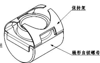
图4 MJ型桶形自锁螺母组件
