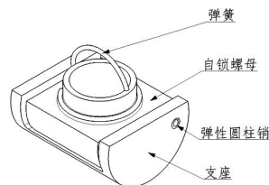
图3 M型桶形自锁螺母组件
