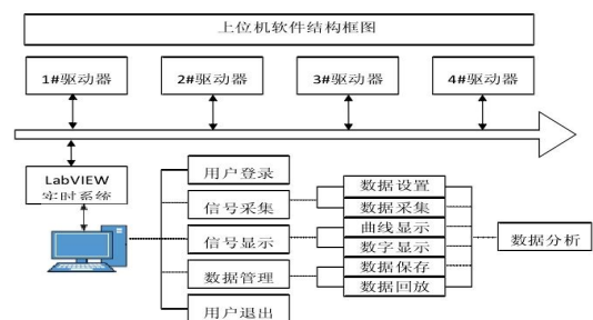
图3 监控系统上位机软件框图
