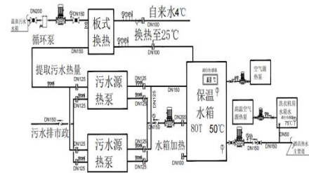
图1 节能改造系统流程图
