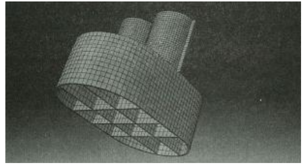
图 1 某港防波堤工程采用的桶式结构
