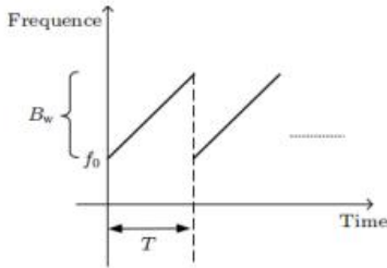
图4 调频连续波信号频域图
