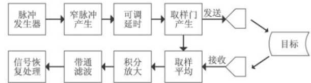
图 2 UWB 雷达系统原理图 [4]
