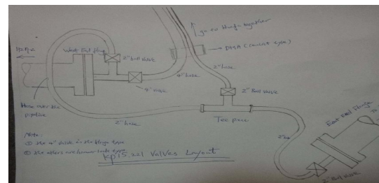
图七 海底管线 KP15 处临时管线配置示意图
