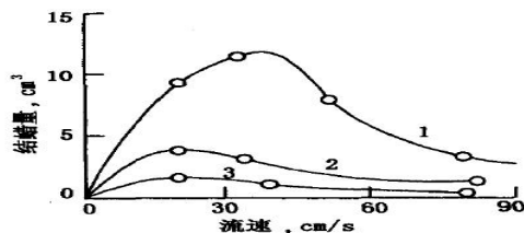
图三 流速与结蜡量的关系
