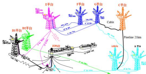
图一 某油田海上石油钻采平台 A.B.C 平台与 FPSO 的位置图
