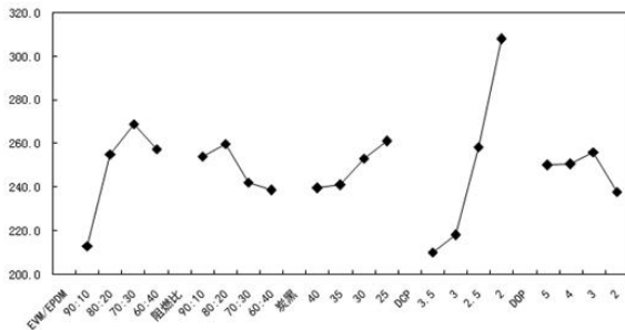
图 3-3 伸长率的效应曲线
