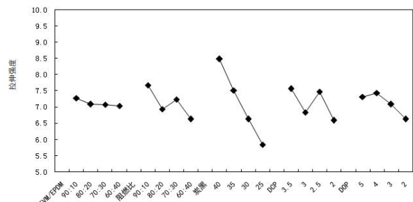
图 3-1 拉伸强度效应曲线
