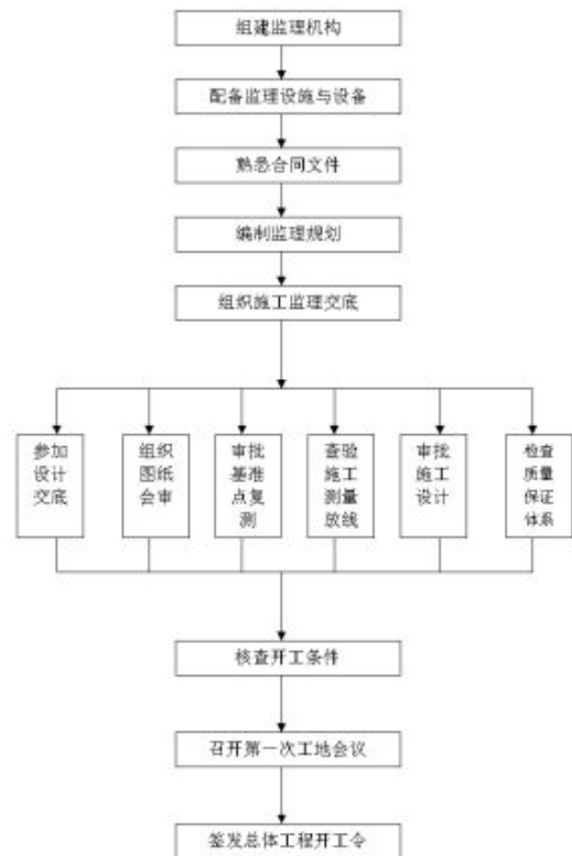
图三所示工程监理准备阶段流程图
