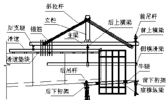
图 1 墩顶施工作业方法
